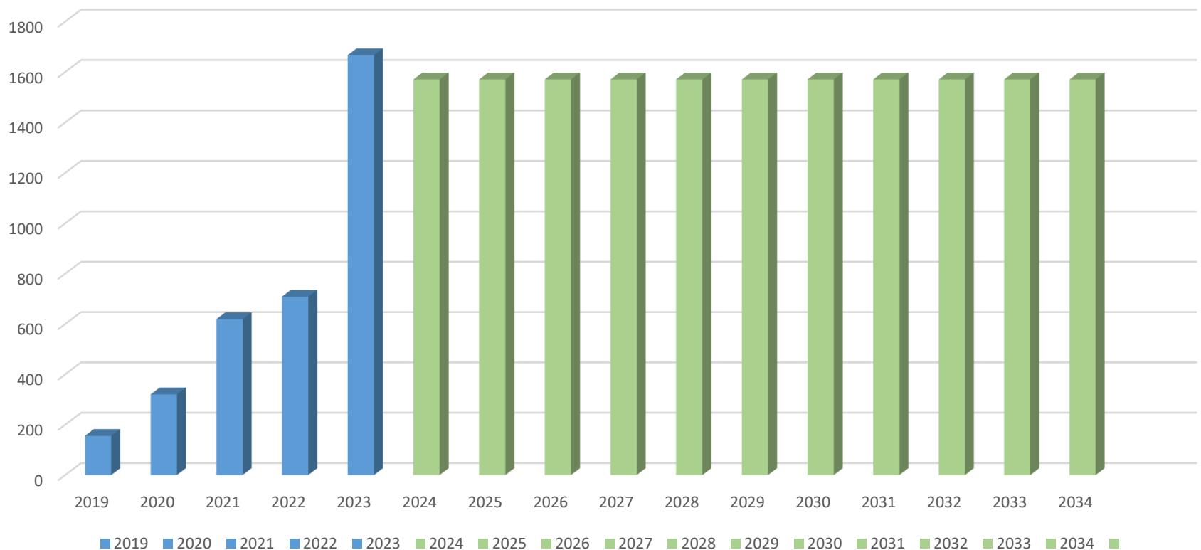
jährlicher Dach-PV-Zubau (in kWp) - bisher / zukünftiges Ziel
